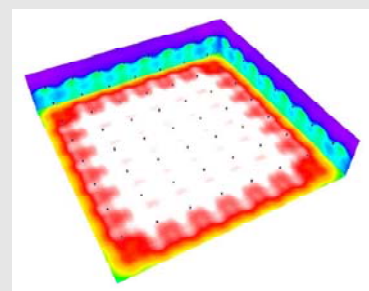
Lysfordeling i 2500m 2 lagerhall, takhøyde 8m (64 stk ZHHB 150W LED, snitt 228 Lux på gulvet )
