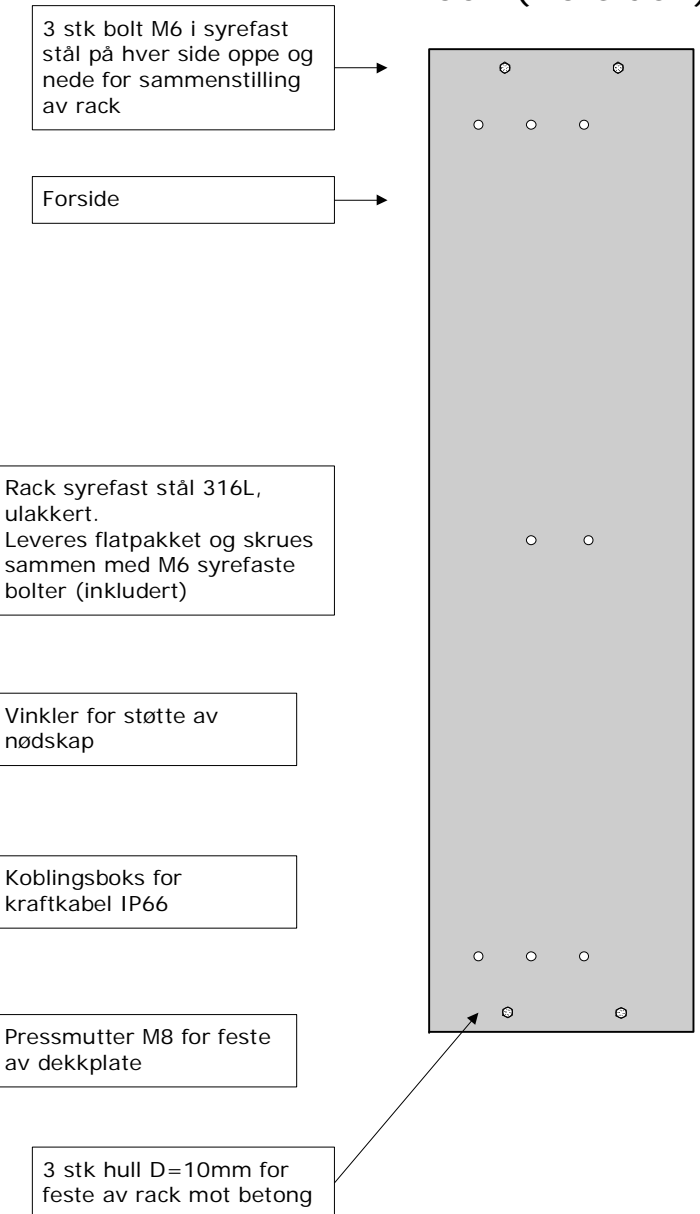
Rack (fra siden)
